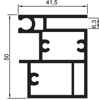
RK-104 Hareketli Dikme/Yatay 1.580 kg/m
