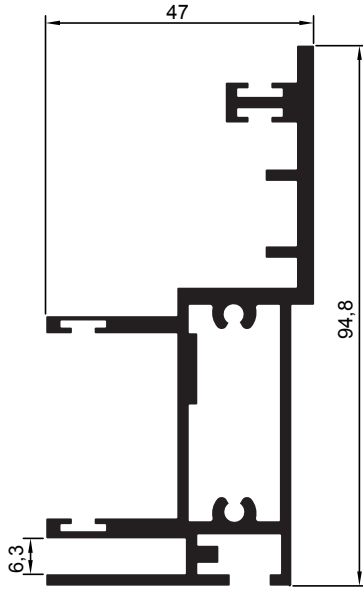
RK-102 Sabit Dikme 2.210 kg/m
