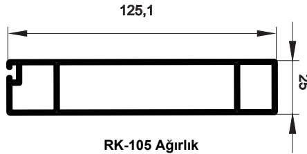
RK-105 Ağırlık 1.406 kg/m
