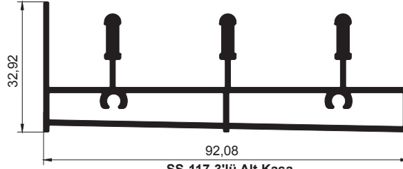
SS-117 3'lü Alt Kasa 1,358 kg/m
