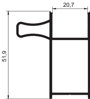
SS-127 ISICAM Tekli Tutamak 0,698 kg/m
