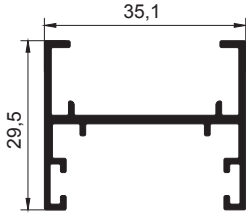
SS-128 Orta Birleşim 0,411 kg/m
