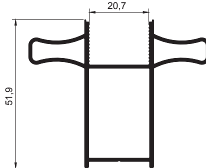
SS-126 ISICAM Çiftli Tutamak 0,920 kg/m
