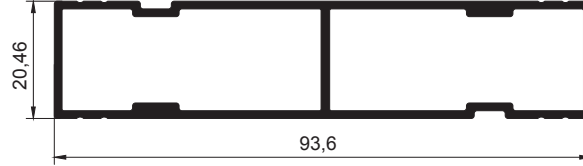
SS-119 3'lü Yan Kasa 0,962 kg/m
