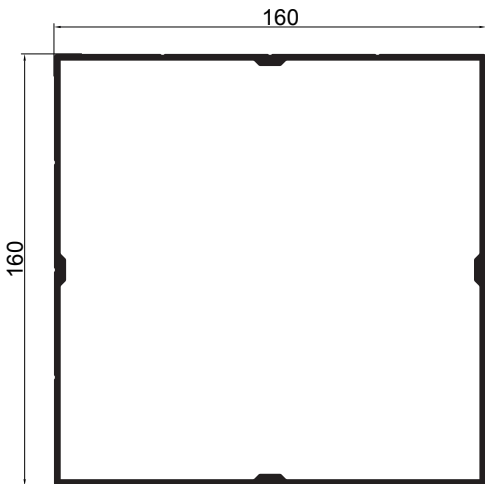
BC-107 160x160 Ayak 4,472 kg/m
