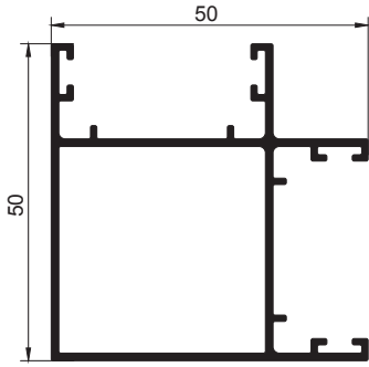
SS-123 90° Köşe Birleşim 0,743 kg/m
