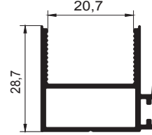
SS-110 Sürme Çekme Baza 0,491 kg/m
