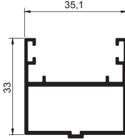
SS-133 Yan Dikme Kanalı 0,513 kg/m
