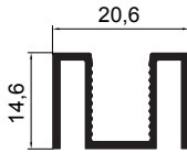
SS-134 Sürme 8mm Adaptör 0,233 kg/m
