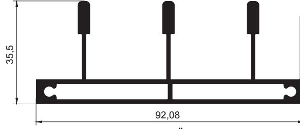
SS-118 3'lü Üst Kasa 1,631 kg/m
