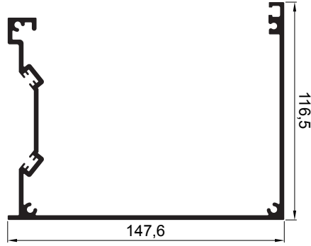
SP-101 Şase 3,335 kg/m
